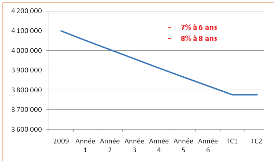
Consommation de l'éclairage de Chartres sur la durée du contrat en KWh
